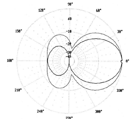
Obr. 5. Azimutální (H) diagram tříprvkové antény ve volném prostoru pro 145,2 MHz (vnější křivka) a elevační diagram (E) (vnitřní křivka). Vnější stupnice 7,39 dBd
