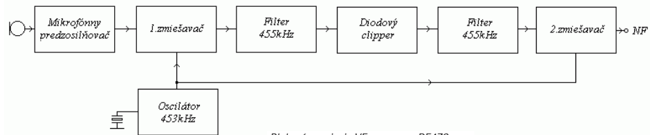
Blokové zapojenie VF procesora DF4ZS
