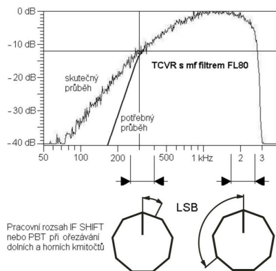
Obr. 2. Kmitočtová nf charakteristika TCVRu i s kvalitním mf filtrem FL80 (9 MHz - 2,3/3,8 kHz - 6/60 dB) nezajistí při poslechu SSB potřebné potlačení kmitočtů pod 300 Hz. V ní dlu si proto pomáhat hornofrekvenční propustí 300 Hz. Jak dolní, tak horní bok filtru FL80 je stejně strmý. Je-li ale kmitočtová osa logaritmická, vypadá průběh nesymetricky. Na knoflíku IF shift nebo PBT vidíme, že na „ucho“ stejně oříznutí nízkých i vysokých kmitočtů je u nízkých kmitočtů stlačeno jen na nepatrné a tedy nepohodlné otočení knoflíkem.
