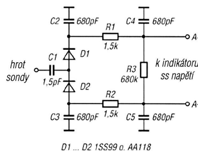
D1 ... D2 1SS99 o. AA118
