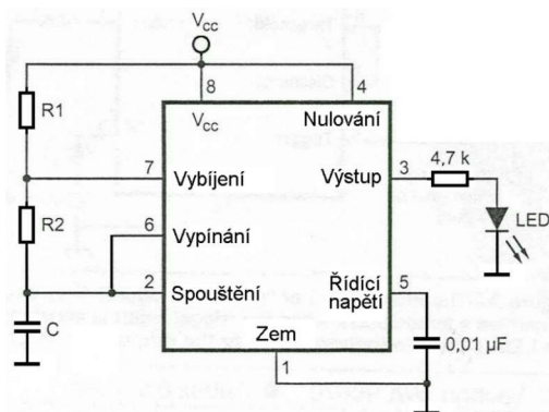
Obr. 3. Astabilní, volně běžící obvod generuje nepřetržitou řadu výstupních pulsů
