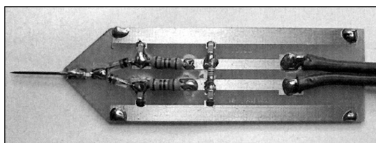
Obr. 1. Téměř dokončená vf sonda před zabudováním do krytu. Nejsou ještě namontovány pružící plechy pro propojení s kovovou trubicou.
