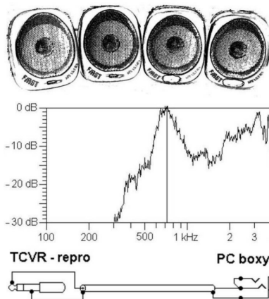
Obr. 3. Kmitočtová charakteristika miniboxů FIRST Austria MS-3043 a zapojení redukce k boxům. Boxy pro svůj tvar nazval Ruda OK1DKR sovími oky. Kmitočtová charakteristika typu „soví oko“ se zdůrazněným vrcholem asi 700 až 800 a 2000 až 2400 Hz se může hodit do SSB závodů, kdy lze čist i stanice nattačené s malým rozestupem. Všimněte si u dvou pravých boxů se zvětšenými basreflexovými otvory 8 x 20 mm ve spodní části. Tím posuneme rezonanci z 720 na 800 Hz, což zvýrazní dále DX SSB i DX CW, zvětší se ale zkreslení pod rezonancí vlivem větší výchylky membrány. Některá zkreslení lze snížit vyzluzněním boxů, stále však zůstává velké zkreslení laciných reproduktorků. Vylepšovat reproboxy k walkmanům tedy nestojí za námahou.
