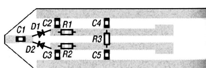
Obr. 3. Na osazovací straně se součástky pájejí přímo na ostrůvků fólie, bez vrtání otvorů
