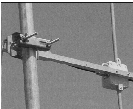
Obr. 2. Upevnění ráhna antény, umožňující posun pro dolaďování antény
