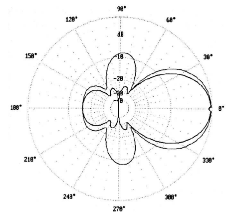
Obr. 6. Azimutální (H) diagram čtyřprvkové antény ve volném prostoru pro 145,0 MHz (vnější křivka) a elevační diagram (E)
